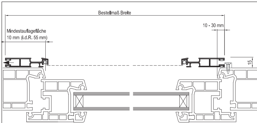
Horizontalschnitt
