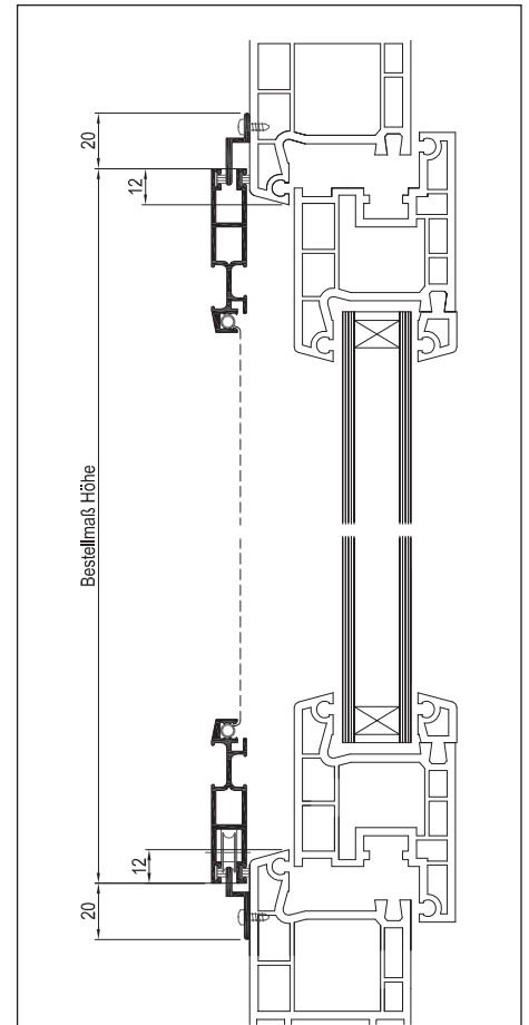
Vertikalschnitt
